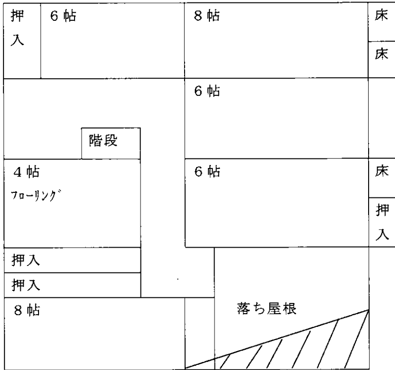
2階
