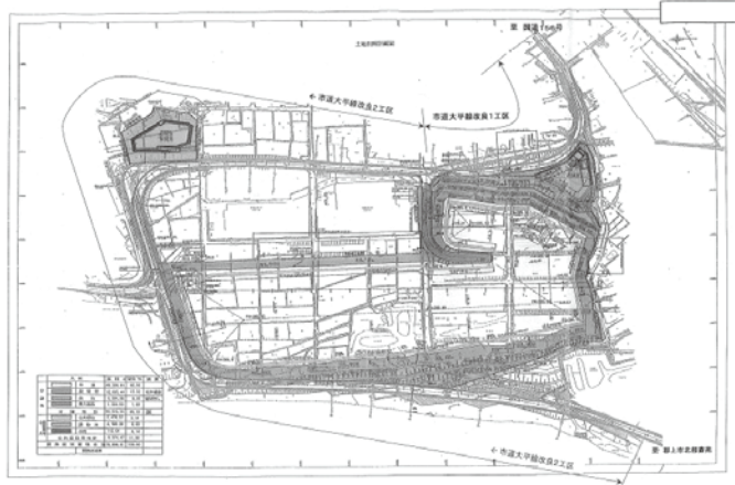
大島工業団地予定平面図
