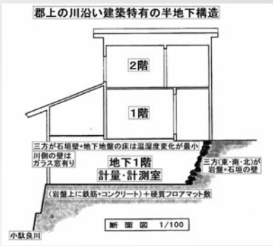
半地下を利用した測定室
