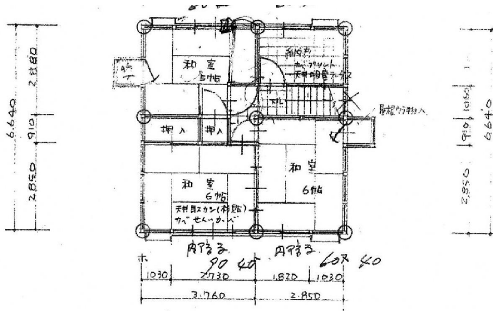
2階平面図 5-1
