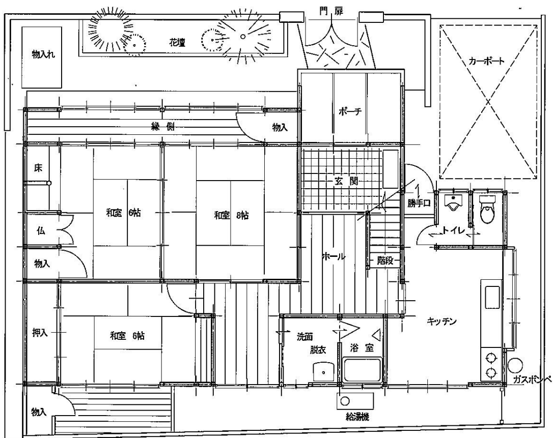
一階平面図
