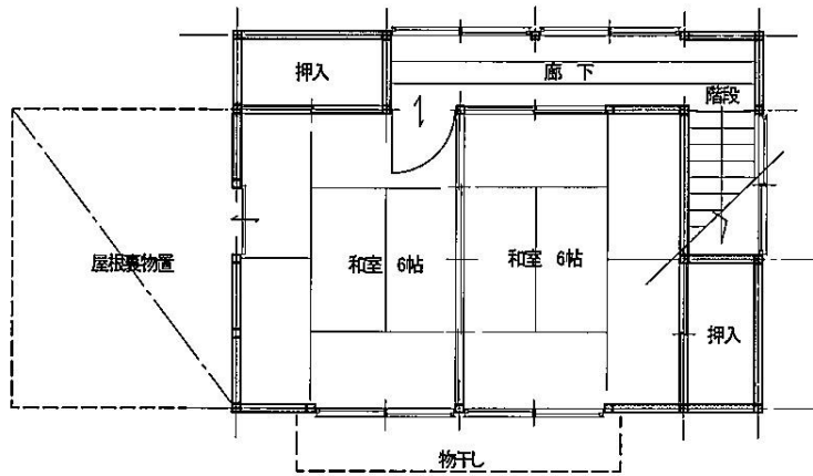
二階平面図
