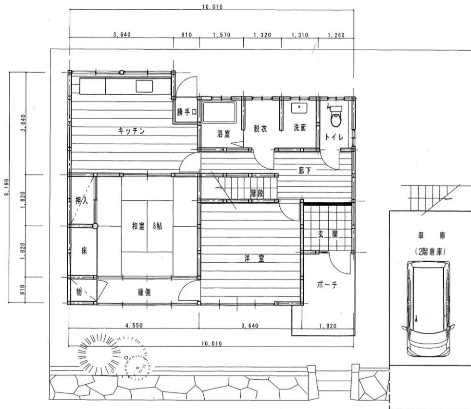
1 階 平 面 図
