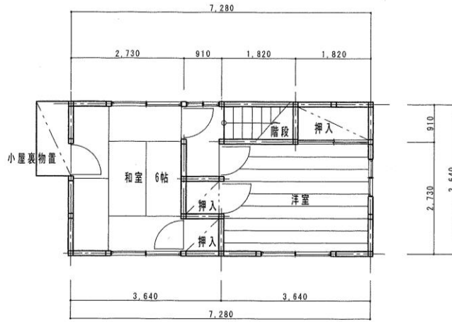
2 階 平 面 図
